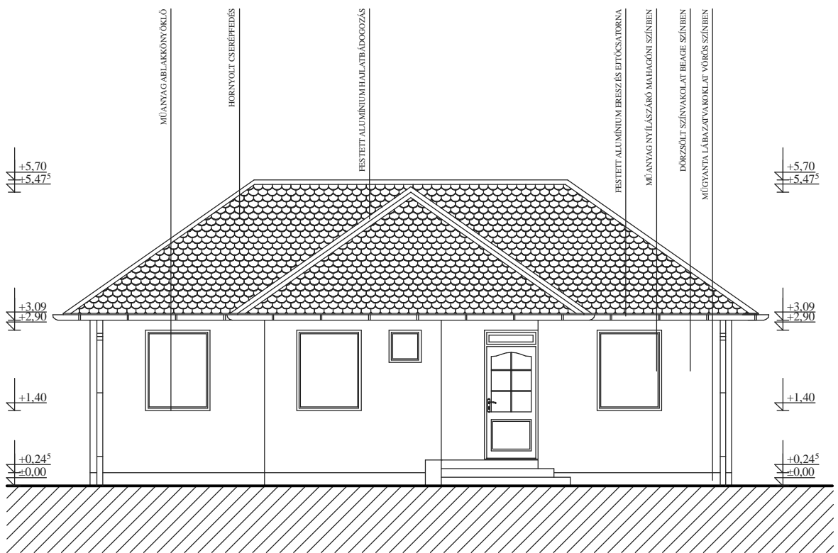
DÉL-KELETI HOMLOKZAT M 1: 100
